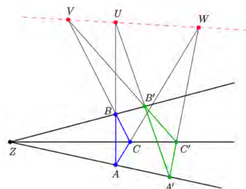
Projektiver Satz von Desargues ( https://commons.wikimedia.org/wiki/User:Ag2gaeh )
