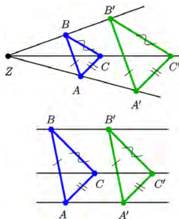
Affine Versionen ( https://commons.wikimedia.org/wiki/User:Ag2gaeh )
